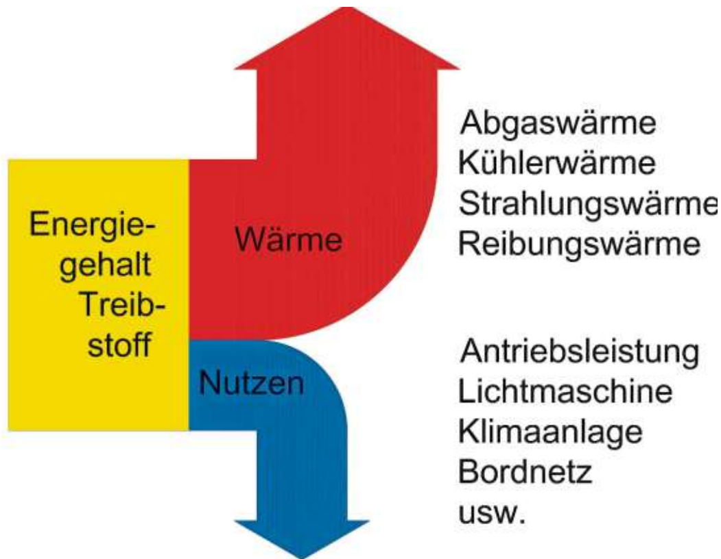
Vereinfachte Schemaskizze: Wirkungsgrad von Wärmekraftmaschinen.
