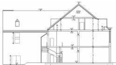
Schnitt A-A
